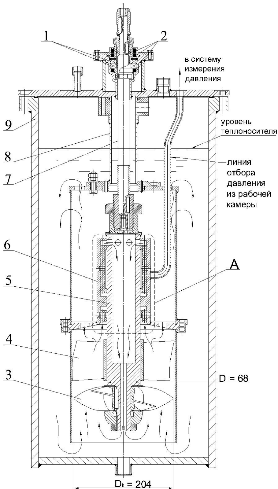
Рис. 1. Схема циркуляции теплоносителя в экспериментальном участке:
