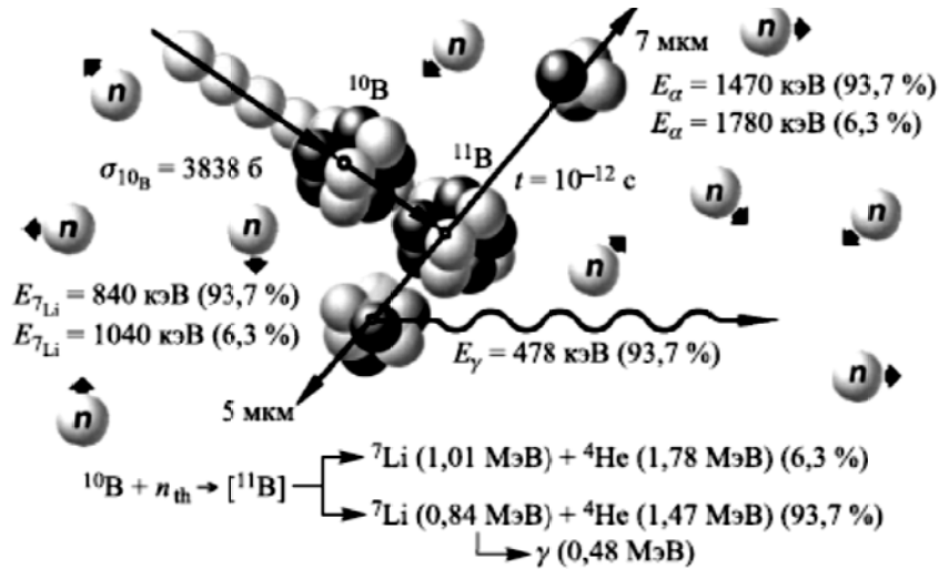
Рис. 1. Схема и характеристики продуктов ядерной реакции
