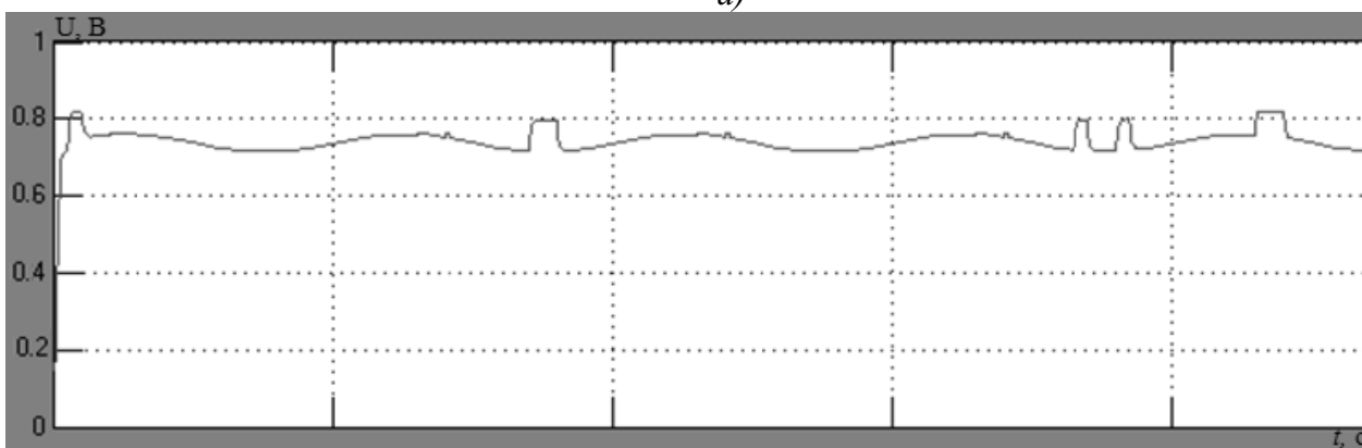
Рис. 5. Результат работы имитационной модели fuzzy-регулятора: а – текущее значение поступающих стоков (уровень резервуара); б – реакция регулятора на изменения уровня поступающих стоков
