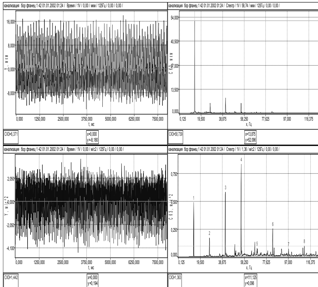
Рис. 6. Исследование резонансных колебаний напорного коллектора КНС
