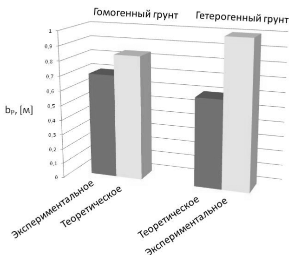
Рис. 7. Гистограмма сравнения теоретических и экспериментальных исследований
