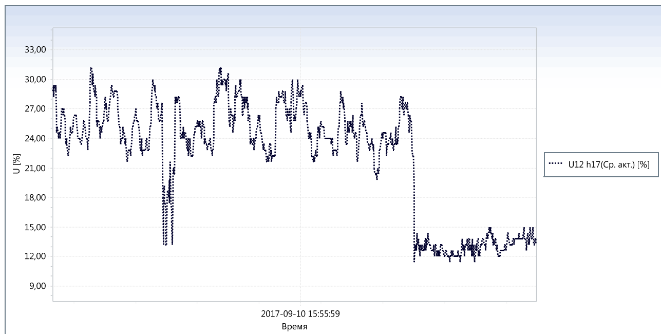
Рис. 6. График изменения семнадцатой гармонической составляющей напряжения
