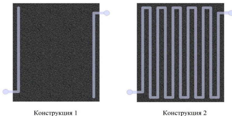
Рисунок 3 – Вид проточных полуячеек различной конструкции
