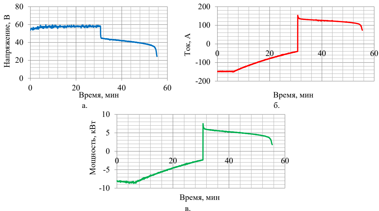
Рисунок 14 – Результаты испытаний ПАКБ при разряде на нагрузку с постоянным сопротивлением
