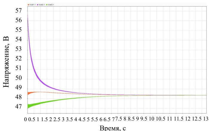
Рисунок 9 – Изменение напряжения ячеек при их параллельном соединении.
