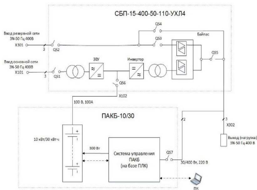
Рисунок 10 – Система бесперебойного питания СБП «ДУБНА»
