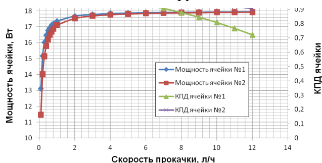
Рисунок 4 – Кривые зависимости мощностей ячеек и их КПД от скорости течения электролита через ячейку
