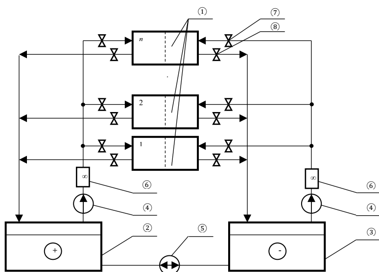
Рисунок 7 – Гидродинамическая схема для подключения нескольких проточных стеков: 1 – стек проточной батареи ( n штук); 2 и 3 – баки с электролитом; 4 – основные насосы прокачки электролита; 5 – балансирующий насос; 6 – датчики расхода электролита; 7 – входные вентили;
