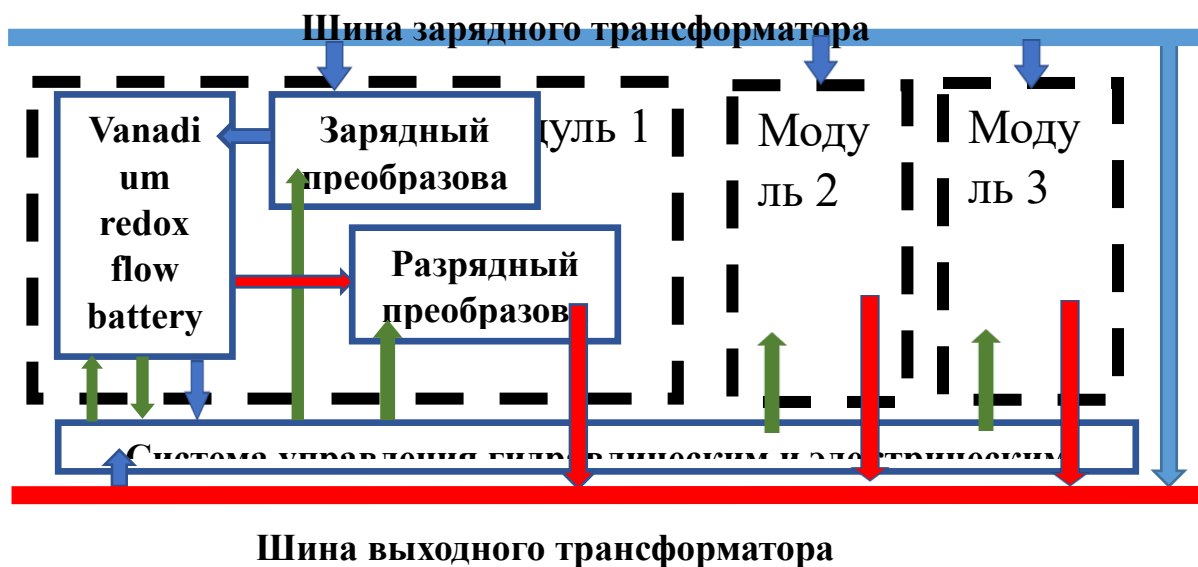
Рисунок 5 - Модульная структура системы включения и управления проточных накопителей
