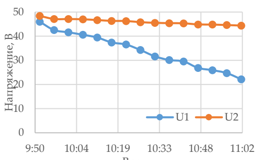
Рисунок 6 – Разрядные характеристики стеков 1 и 2.
