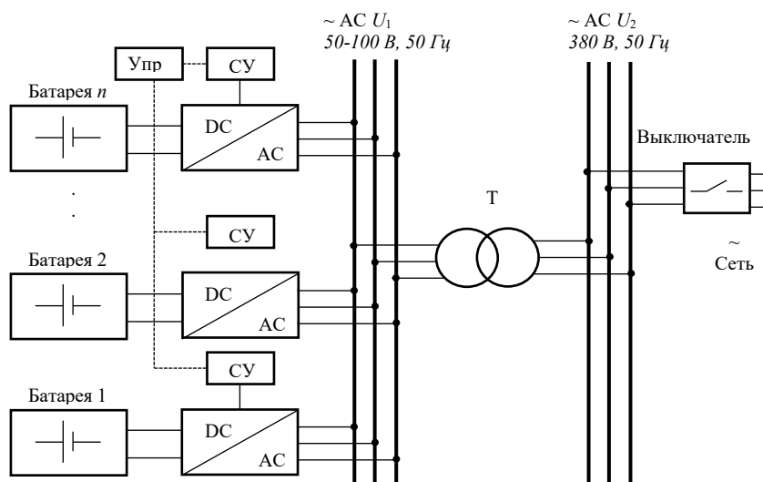
Рисунок 8 – Функциональная схема объединения стеков и их преобразователей на параллельную работу.
