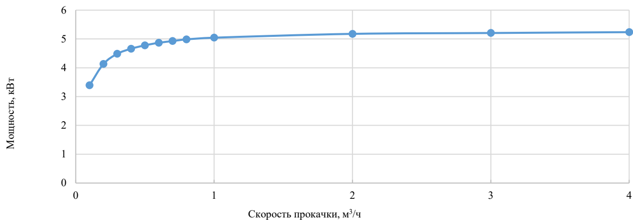
Рисунок 11 – Зависимость мощности стека от скорости течения электролита.
