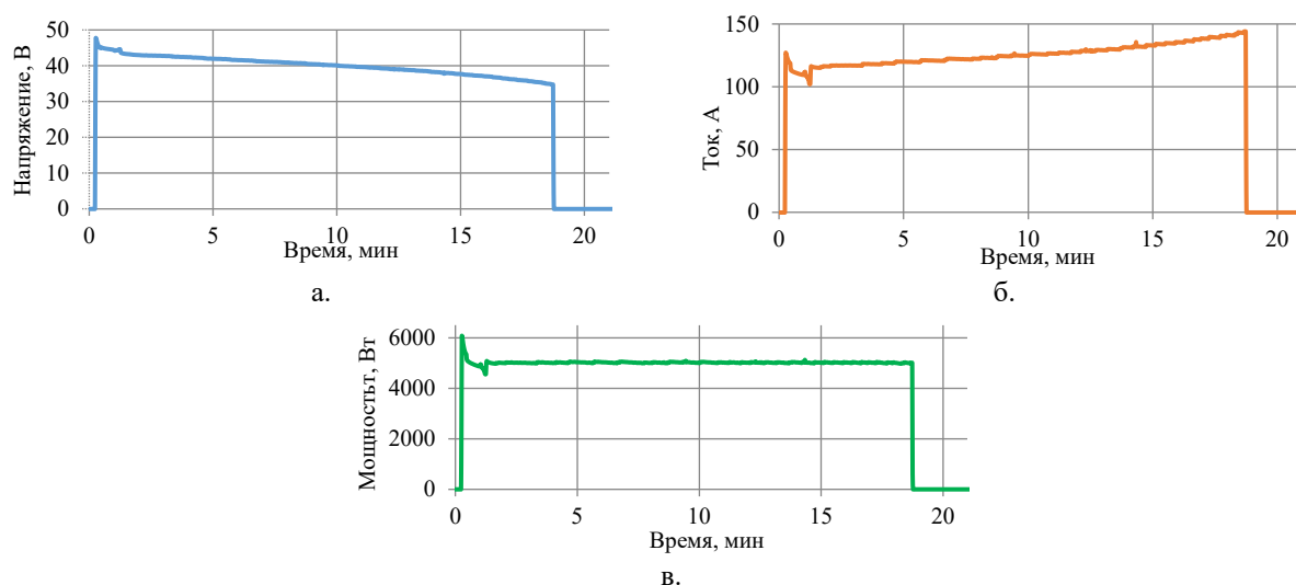
Рисунок 15 – Результаты испытаний ПАКБ при разряде на нагрузку с постоянной мощностью
