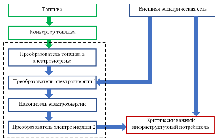
Рисунок 2 – Структура локальных источников на основе преобразователей топлива.
