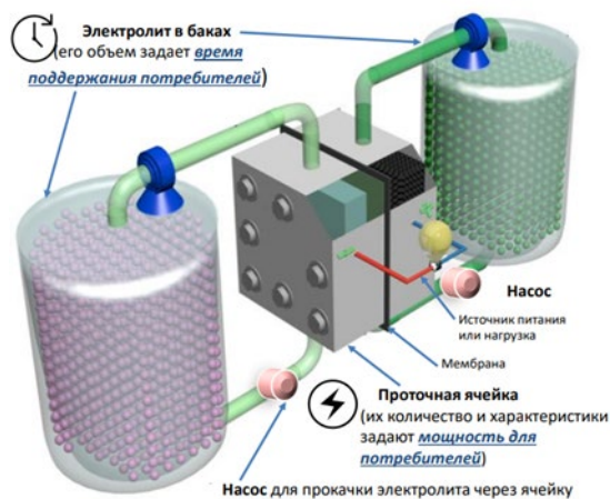
Рисунок 1 – Проточная ячейка
