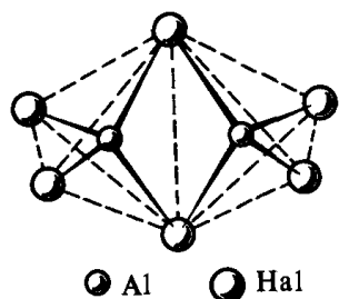
Р и с. 194. Строение молекулы \text{Al}_2\text{Hal}_6
