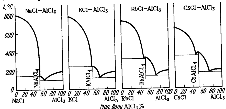
Р и с. 134. Диаграмма плавкости систем MCl - AlCl 3
