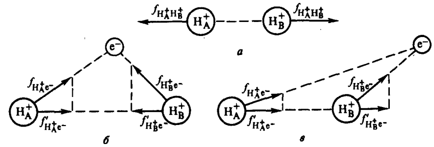
Р и с. 18. Силы взаимодействия между протонами и электроном в молекулярном ионе \text{H}_2^+
