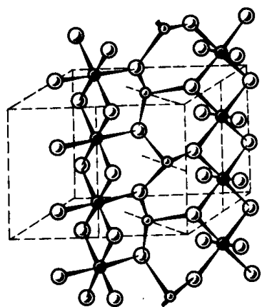
Р и с. 181. Структура сурика \text{Pb}_3\text{O}_4 ( \text{Pb}_2\text{PbO}_4 )
