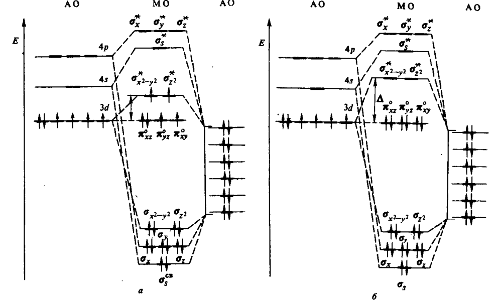
Рис. 218. Схема распределения валентных электронов по молекулярным орбиталям:
