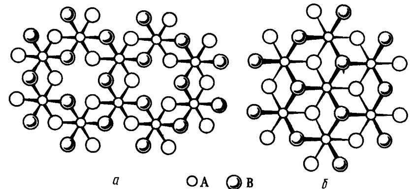
Р и с. 236. Структура слоя, образованного октаэдрическими структурными единицами \text{AB}_6 , соединения типа \text{AB}_3 (а) и соединения типа \text{AB}_2 (б)
