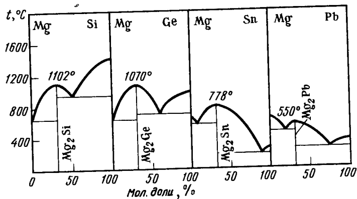
Рис. 180. Диаграмма плавкости систем \text{Mg—Si} , \text{Mg—Ge} , \text{Mg—Sn} , \text{Mg—Pb}
