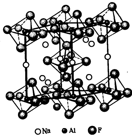
Р и с. 195. Структура криолита \text{Na}_3\text{AlF}_6
