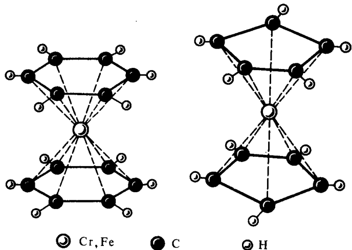
Р и с. 224. Строение дихлорхрома \text{Cr}(\text{C}_6\text{H}_6)_2 и ферроцена \text{Fe}(\text{C}_5\text{H}_5)_2
