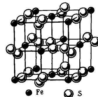
Р и с. 155. Кристаллическая решетка пирита FeS_2
