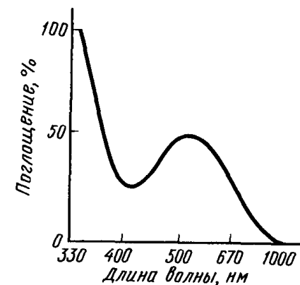
Р и с. 223. Спектр поглощения комплекса [\text{Ti}(\text{OH}_2)_6]^{3+}
