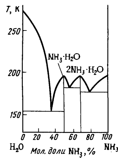
Рис. 158. Диаграмма состояния системы \text{H}_2\text{O} - \text{NH}_3
