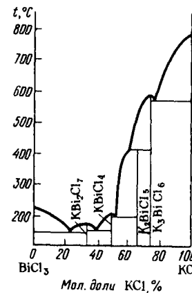
Рис. 170. Диаграмма плавления системы \text{BiCl}_3 — \text{KCl}
