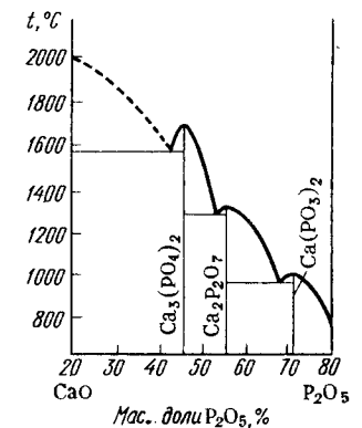
Рис. 167. Диаграмма плавления системы CaO - P_2O_5
