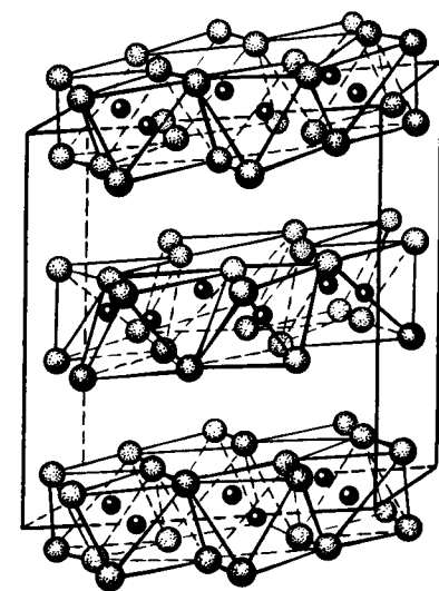
● Al ● OH
