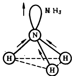
Р и с. 55. Сложение электрических моментов диполя связывающих и несвязывающих электронных пар молекул NH 3 и NF 3
