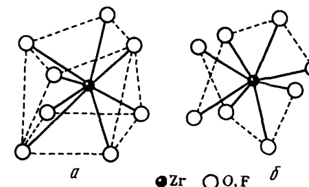
Рис. 227. Взаимное расположение атомов ZrO 2 с примесью HfO 2 в восьмивершинниках оксо- (а) и названных фианитами . Последние имеют высокий показатель преломления, отличаются высокой твердостью, прочностью, исключительной химической стойкостью. Их применяют в технике и для изготовления украшений.
