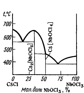
Р и с. 231. Диаграмма плавления системы \text{CsCl} - \text{NbOCl}_3
