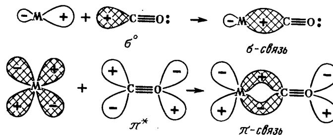
Р и с. 232. Схема образования \sigma - и \pi -связей М – CO в карбонилах d -элементов: заштрихованные орбитали содержат электроны; незаштрихованные — свободны
