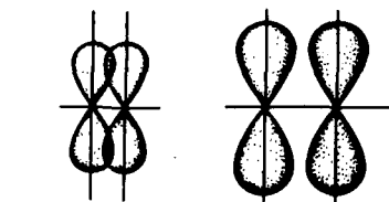
Р и с. 147. Влияние междерного расстояния на степень перекрывания p\pi-p\pi -связей
