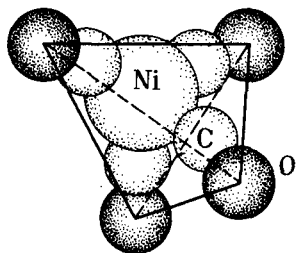
Рис. 242. Строение молекулы тетракарбонила никеля Ni(CO) 4
