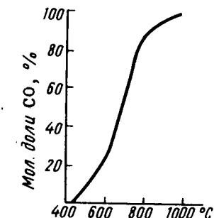
Рис. 177. Влияние температуры на состояние равновесия CO_2(г) + C(к) \rightleftharpoons 2CO(г) .
