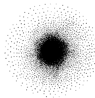
Рис. 2. Электронное облако
