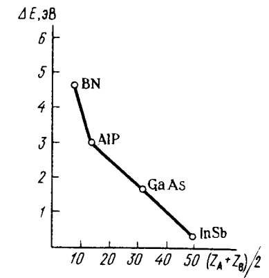
Р и с. 199. Зависимость ширины запрещенной зоны \Delta E в соединениях типа A^{III}B^V от среднеарифметического атомного номера
