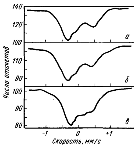
Р и с. 241. \gamma -Спектры берлинской лазури (а) и турбуллевой сини (б) и солей KFe[Fe(CN)_6] и KFe_2[Fe(CN)_6] (в)
