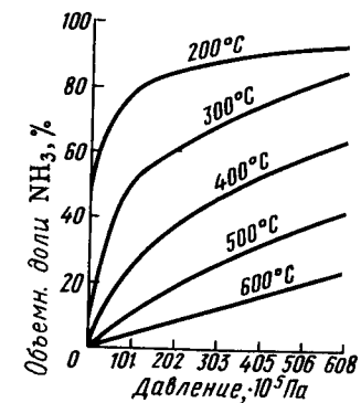
Р и с. 159. Равновесная концентрация аммиака в азотодородной смеси ( 3\text{H}_2 + \text{N}_2 ) как функция давления и температуры
