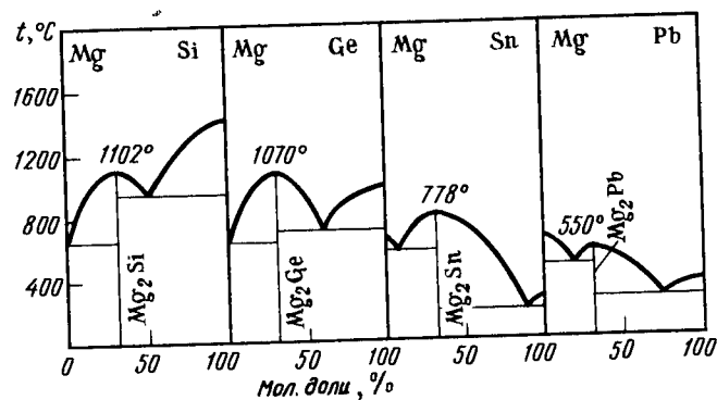
Рис. 180. Диаграмма плавкости систем Mg — Si, Mg — Ge, Mg — Sn, Mg — Pb
