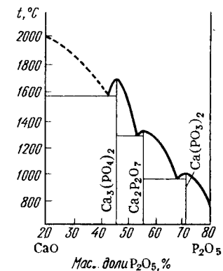
Рис. 167. Диаграмма плавления системы CaO - P_2O_5
