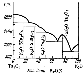
Р и с. 229. Диаграмма плавкости системы Ta 2 O 5 - K 2 O
