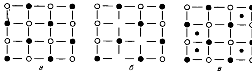
Р и с. 137. Дефекты кристаллической решетки соединения АВ:
