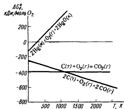
Р и с. 113. Зависимость \Delta G_f^0 ряда оксидов от температуры
