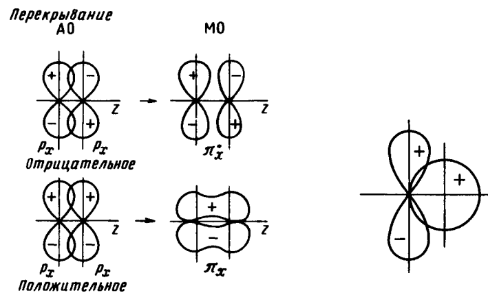
Р и с. 25. Схема образования из p_x -атомных орбиталей связывающей \pi_x и разрыхляющей \pi_x^* молекулярных
