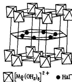
Р и с. 202. Структура бишофита MgCl_2 \cdot 6H_2O
