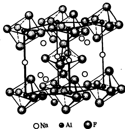
Рис. 195. Структура криолита Na_3AlF_6
