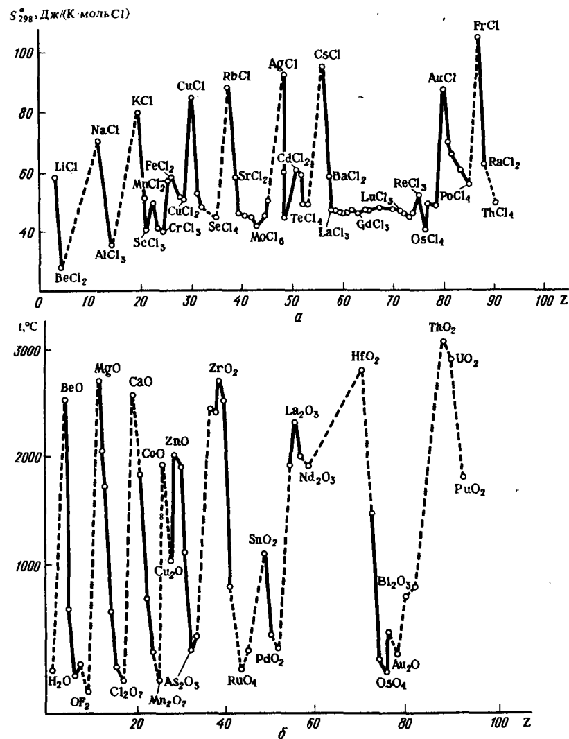
Р и с. 131. Зависимость свойств бинарных соединений от атомного номера элемента с положительной степенью окисления:
