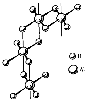
Р и с. 196. Фрагмент структуры гидроксида алюминия (\text{AlH}_3)_n
