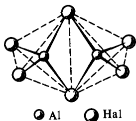
Рис. 194. Строение молекулы Al_2Hal_6
