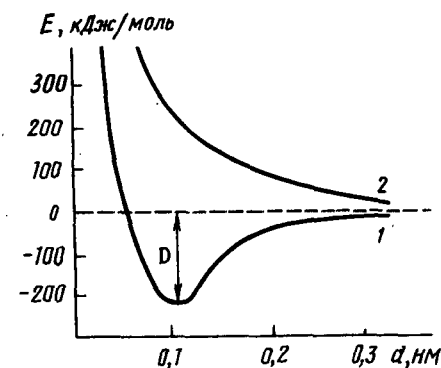
Р и с. 20. Зависимость потенциальной энергии молекулярного иона \text{H}_2^+ при нахождении электрона в связывающей (кривая 1) и разрыхляющей (кривая 2) области
