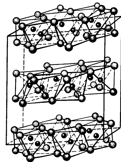
● Al ● OH
