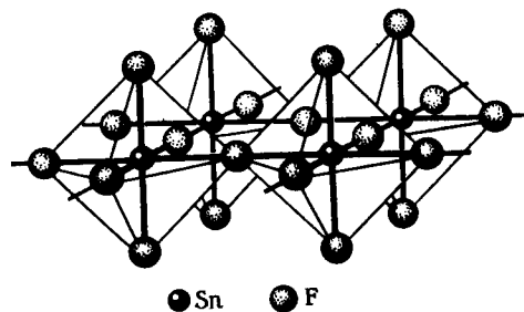
Р и с. 182. Структура SnF 4
