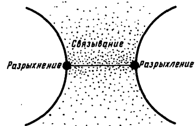
Р и с. 19. Области связывания и разрыхления в молекулярном ионе \text{H}_2^+
