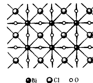
Рис. 171. Структура слоя кристаллического \text{BiOCl} : атомы \text{O} и \text{Cl} лежат соответственно выше и ниже плоскости из атомов \text{Bi}
