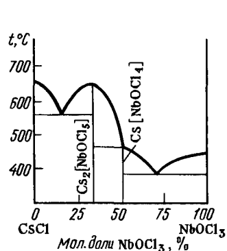
Рис. 231. Диаграмма плавления системы \text{CsCl} - \text{NbOCl}_3
