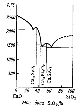
Рис. 178. Диаграмма плавления системы \text{CaO}-\text{SiO}_2
