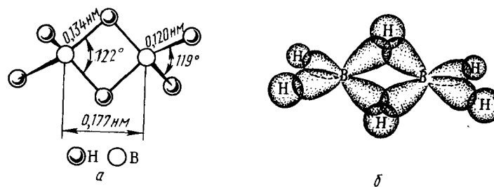
Рис. 185. Строение (а) и схема перекрывания атомных орбиталей (б) в молекуле B_2H_6
