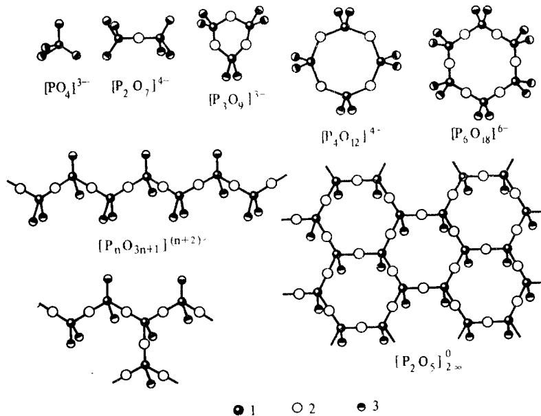
Рис. 166. Структура оксофосфат (V)-ионов и слоистой модификации P_2O_5 :
