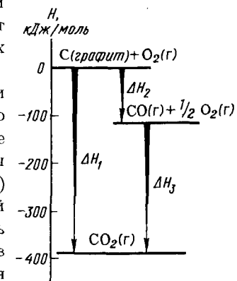
Рис. 109. Энтальпийная диаграмма окисления графита
