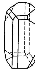
\beta -S
