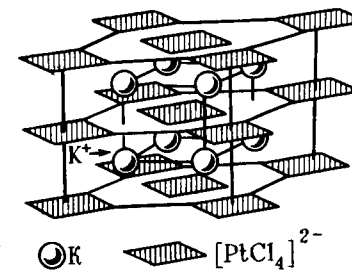
Р и с. 247. Структура \text{K}_2[\text{PtCl}_4]
