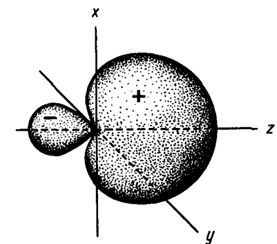
Р и с. 47. Форма sp -гибридной орбитали
