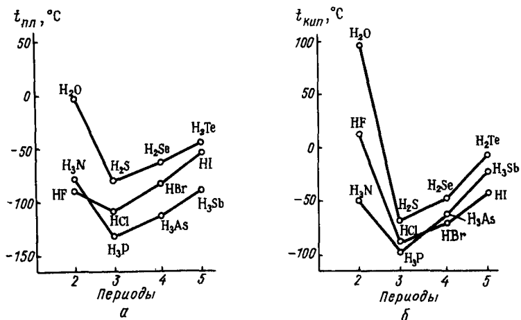
Р и с. 148. Температуры плавления (а) и кипения (б) водородных соединений р-элементов VII, VI, V групп
