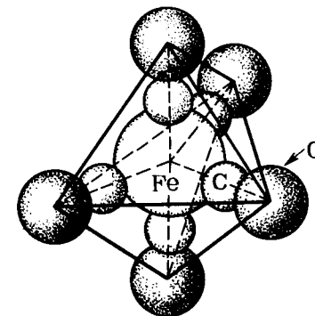
Рис. 240. Структура молекулы пентакарбонила железа \text{Fe}(\text{CO})_5
