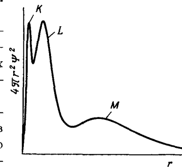
Рис. 11. Распределение электронной плотности в атоме аргона
