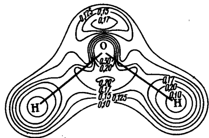
Рис. 17. Распределение электронной плотности в молекуле воды
