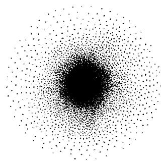
Рис. 2. Электронное облако
