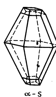
\alpha -S
