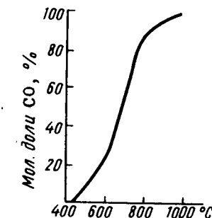
Рис. 177. Влияние температуры на состояние равновесия CO_2(г) + C(к) \rightleftharpoons 2CO(г) .
