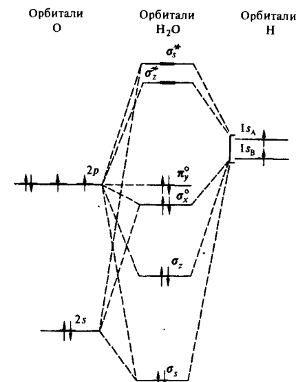
Рис. 151. Энергетическая диаграмма орбиталей молекулы H_2O
