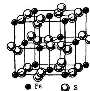
Р и с. 155. Кристаллическая решетка пирита FeS_2
