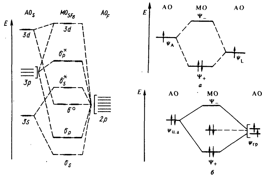
Р и с. 145. Энергетическая диаграмма орбиталей для двухэлектронного (а) и трехэлектронного четырехэлектронного взаимодействия (б)
