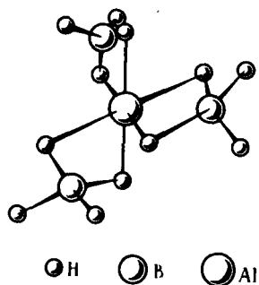
Р и с. 197. Структура \text{Al}(\text{BH}_4)_3
