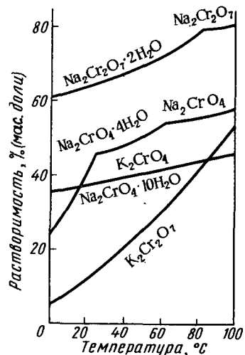
Рис. 238. Растворимость хроматов (VI) и дихроматов (VI) калия и натрия
