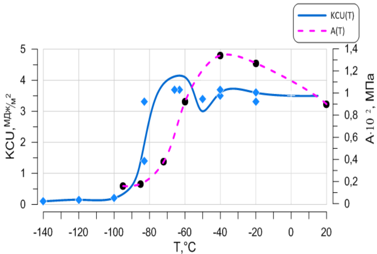
Рис. 1. Зависимость KCU (T) и A (T) армко-железа при отпуске 450 °C
