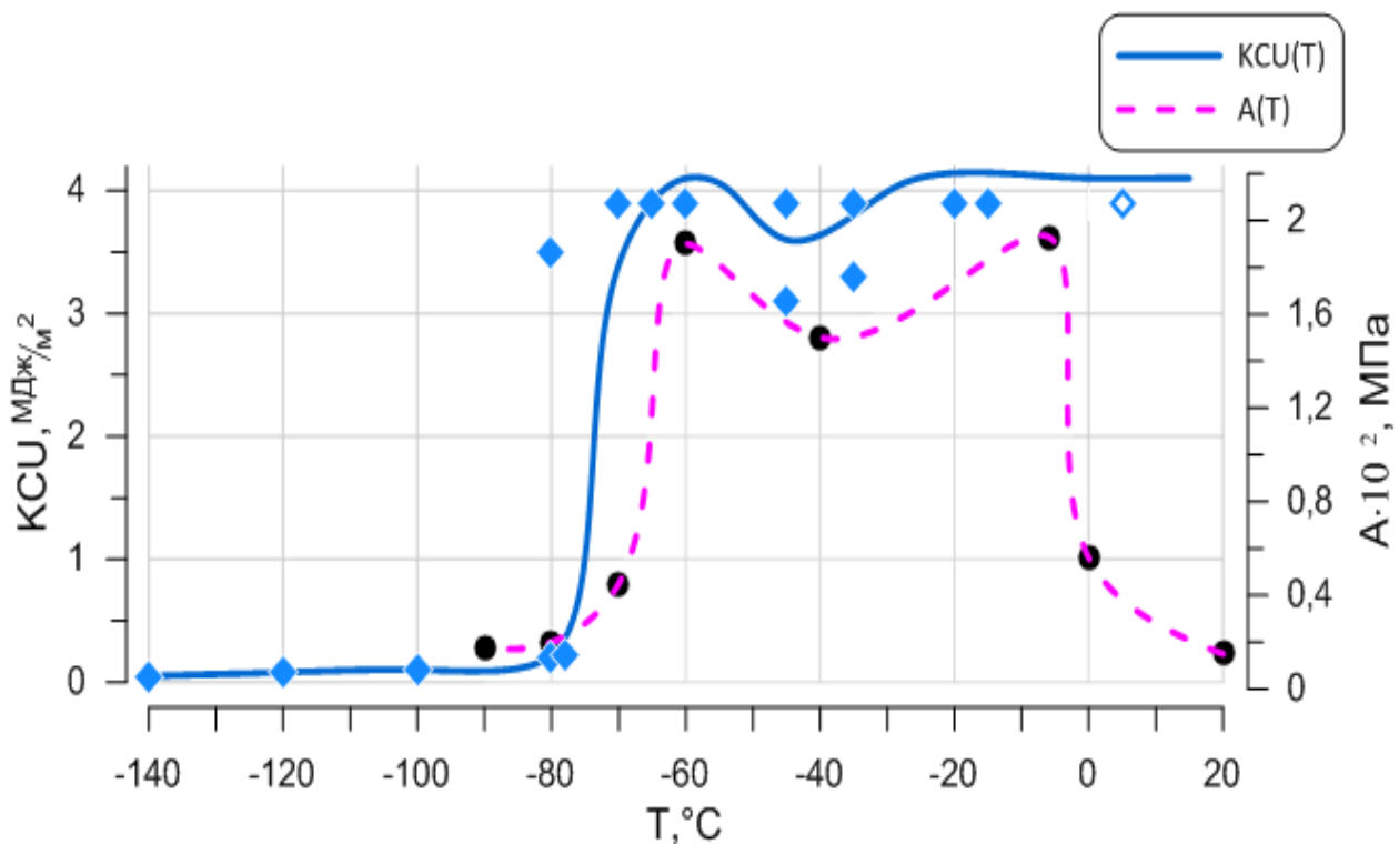
Рис. 2. Зависимость KCU (T) и A (T) армко-железа при отпуске 650 °C
