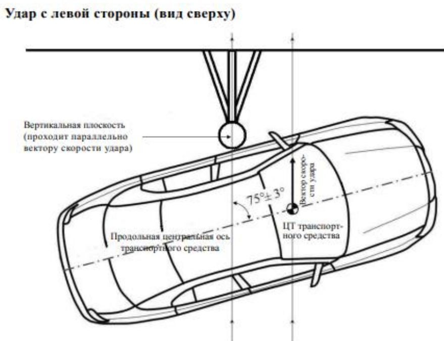
Рис. 1. Испытания по Правилу ЕЭК ООН №135
