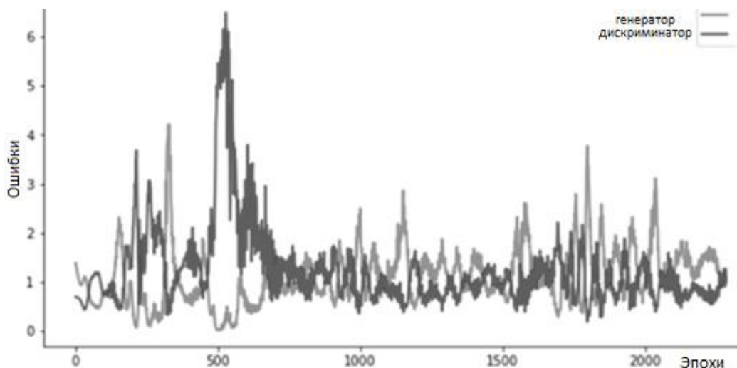
Рис. 6. График обучения
