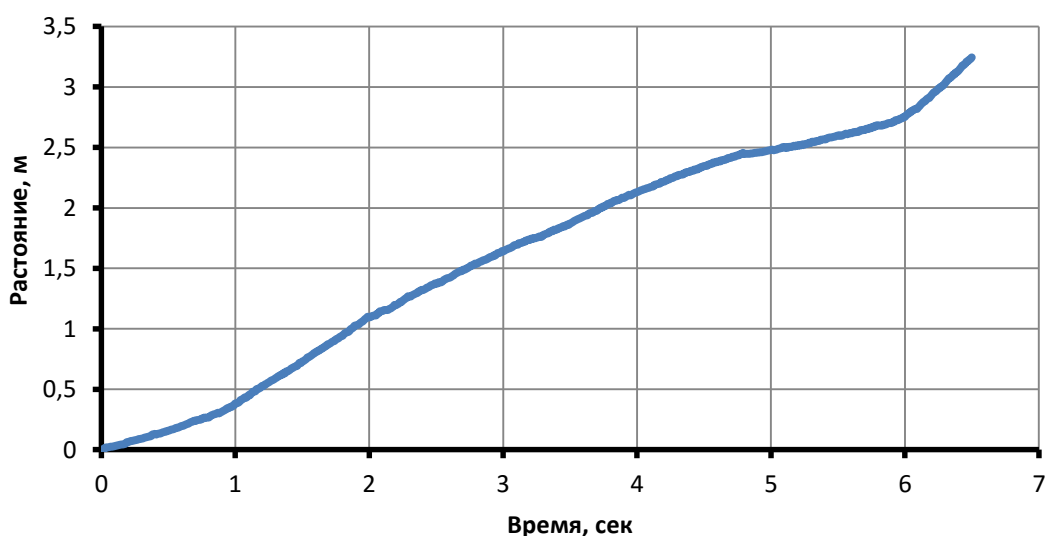
Рис. 8. Отклонение траектории
