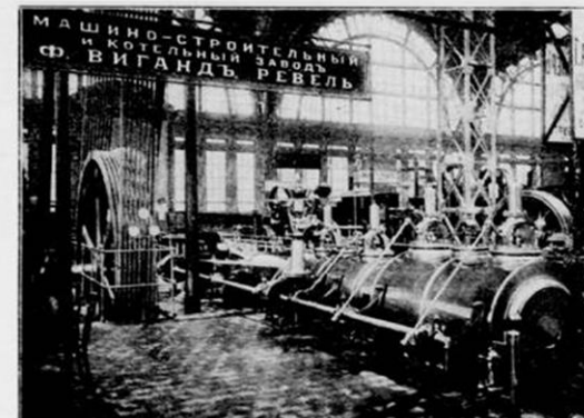
Кохпаудъ-вентиляціонная паровая машина, изготовленная фирмой Фр. Вигандъ въ Ревелѣ.
