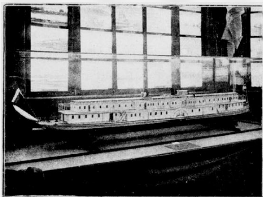
Модель парохода „Святославъ“.
