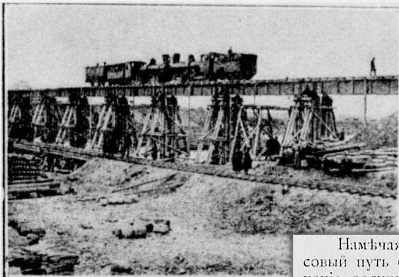
Мостъ на р. Вологдѣ.
