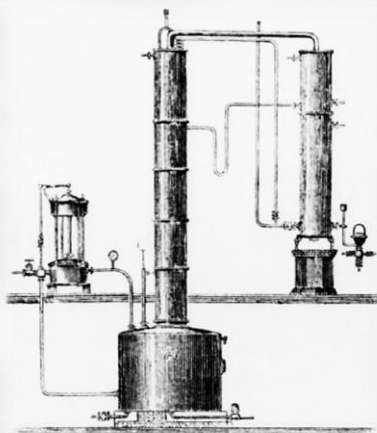
Ректификаціонный аппаратъ.
