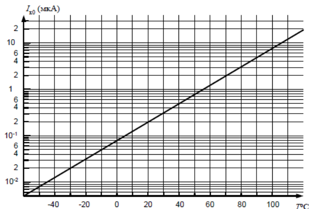
Зависимость обратного тока коллектора от температуры
