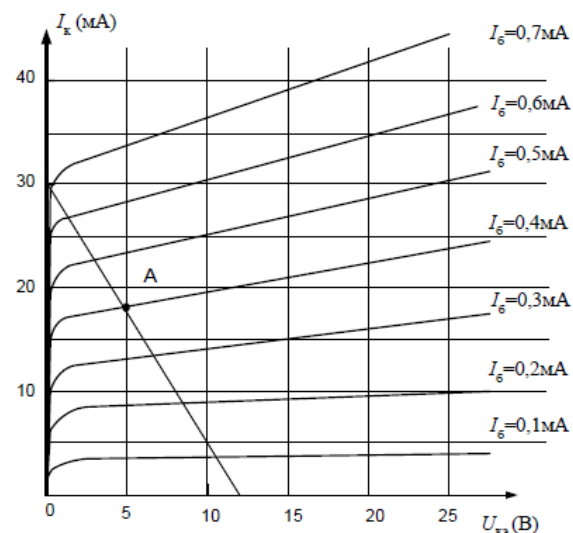
Выходные характеристики транзистора КТ312Б
