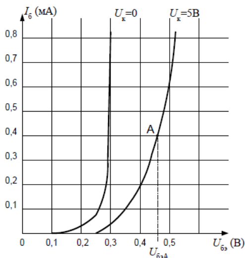
Входные характеристики транзистора КТ312Б
