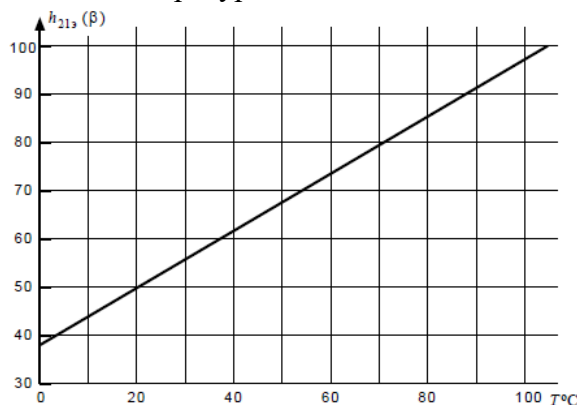
Зависимость коэффициента усиления тока базы от температуры
