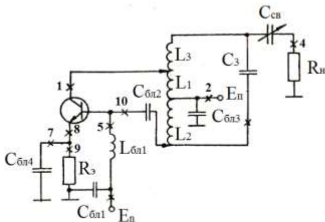
Рис. 2. Схема автогенератора (индуктивная трёхточка)
