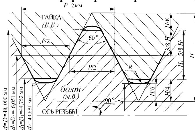
Рис. 3 Эскиз резьбового соединения:
