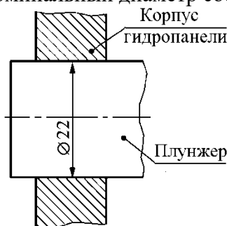
Рис. 3. Схема соединения «плунжер-отверстие» в корпусе гидропанели
