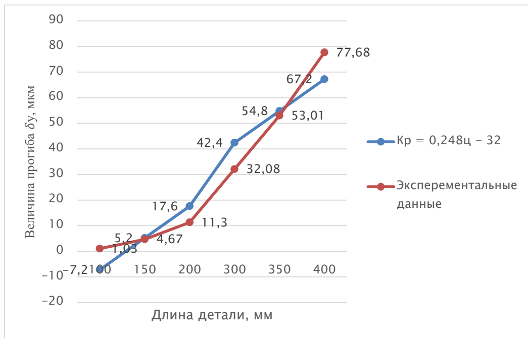
Рис. 3. Наложение экспериментальных данных на расчетную функцию K_p = 0,248z - 32
