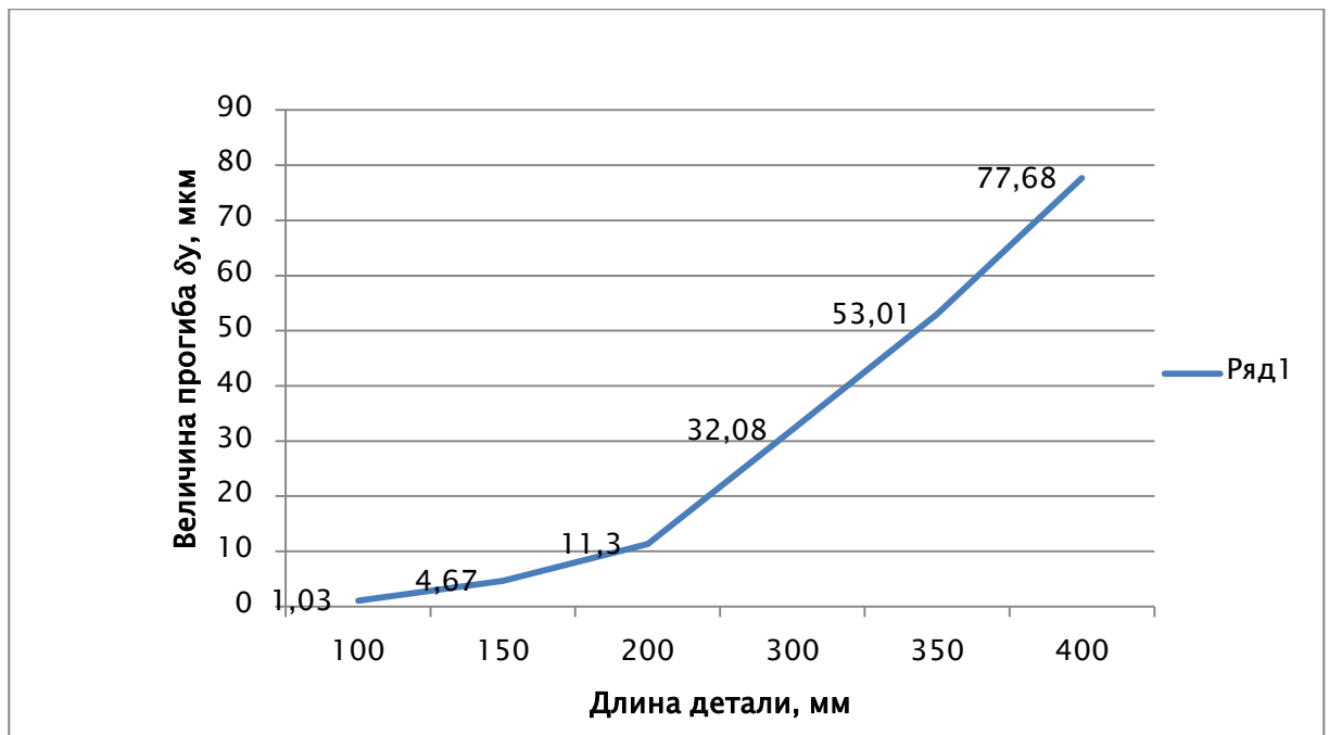
Рис. 1. Диаграмма экспериментальных данных
