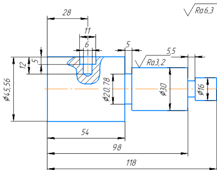
Рисунок 1 – Чертеж детали
