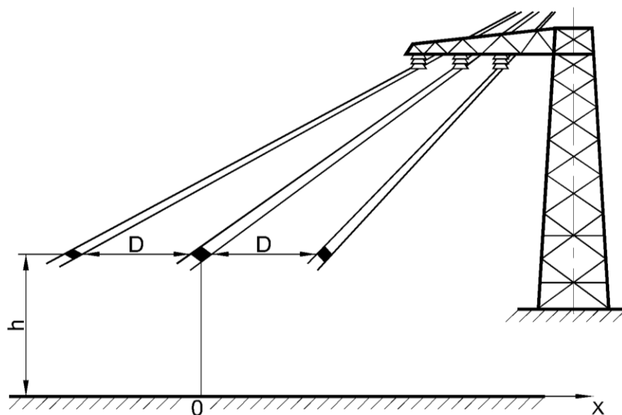
Рис. 1. Схема воздушной линии
