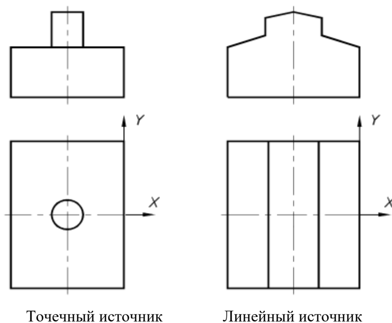
Рис.2 Источники технологических выбросов: а – точечный источник,
